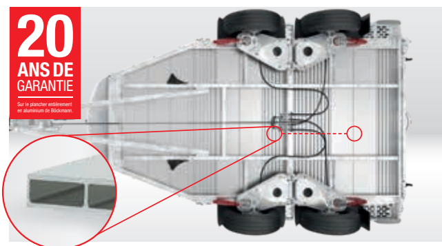
Robuste, imputrescible et conçu pour des charges élevées grâce au plancher en aluminium massif à profilés fermés sous les pieds des chevaux ainsi qu'à la construction du châssis avec longerons et cadre en acier galvanisé à chaud.
