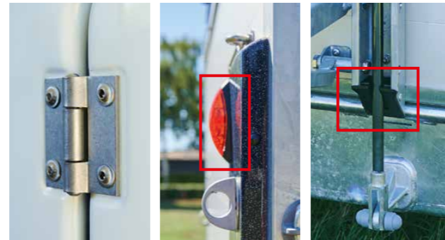
Absence absolue de coins et d'arêtes avec des charnières arrondies et des caches en plastique au niveau des montants profilés en acier et aux extrémités des renforts arrières.
