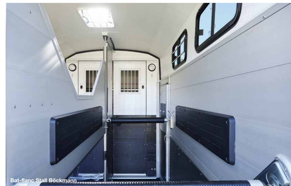
Bat-flanc Böckmann
