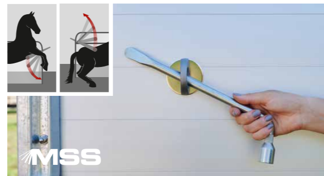
Déblocage rapide en cas d'urgence grâce au système anti-panique éprouvé des barres de sécurité Multi Safe (MSS) Peut être débloqué à l'avant et à l'arrière. La clé démonte-roues fait partie de l'équipement de série.
